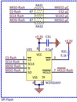
SPI Flash
